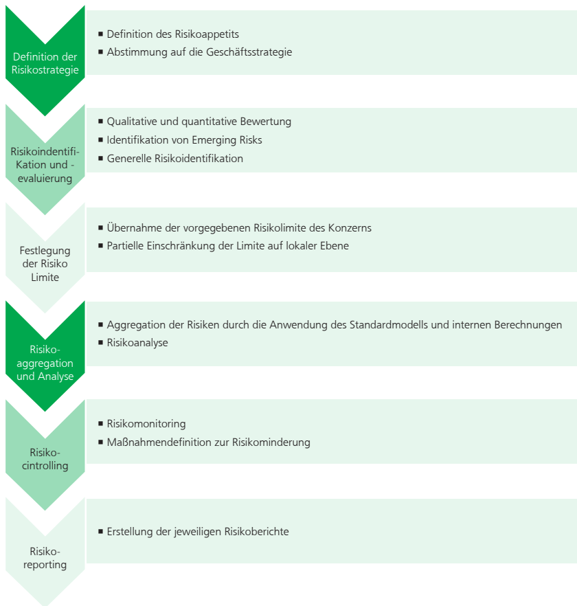
Abbildung 15: Risikomanagementprozess
